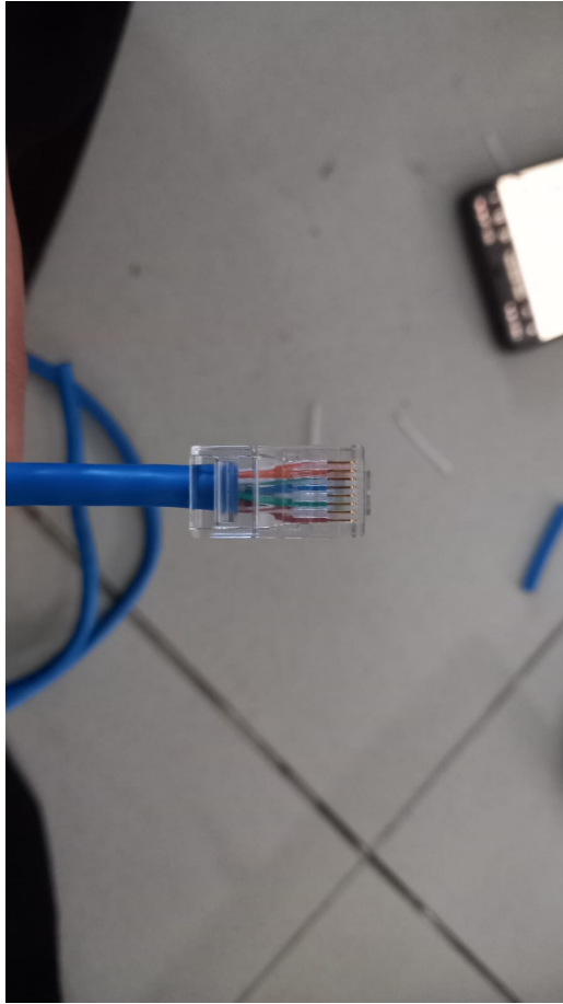
Gambar 19: Dokumentasi hasil akhir kabel LAN setelah proses crimping selesai dilakukan.
